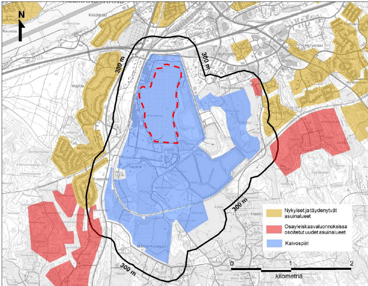
Kuva 51. Kaivospiiri ja tärinäalue. Geomatti Oy 2016
