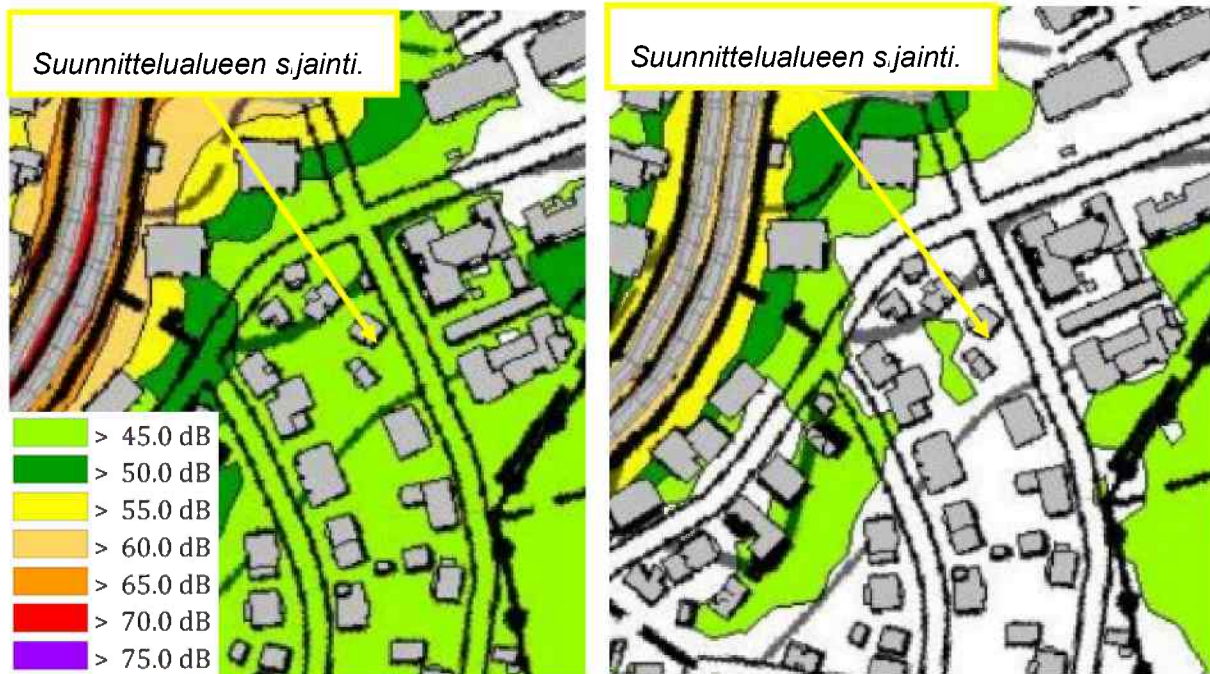
Kuva 17 Lappeenrannan keskustajaman meluselvitys: Ennustetilanne v. 2040. Vasemmalla päiväjän keskiäänitasot LAeq 7-22. Oikealla yöajan keskiäänitasot LAeq 22-7.
