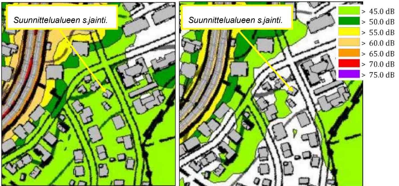
Kuva 12. Vasemmalla nykytilanteen v. 2020 päiväjän keskiäänitasot ja oikealla nykytilanteen v. 2024 päiväjän keskiäänitasot. (Lähde Lappeenrannan seudun ympäristötoimen meluselvitys 2021).
